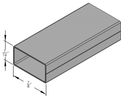
7/16 X 7/8 SDL GRILLE BAR - 152" SKU: S-137 Category: Grille Bar UMO: FT
