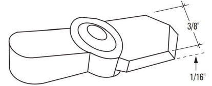
TURN CLIP 1/16" STEP - NYLON
