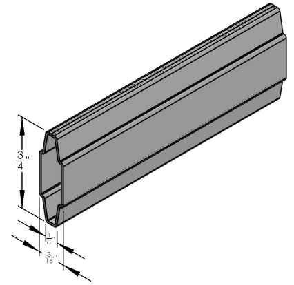
5.5MM X 18MM CONTOUR BAR - 12'8"
