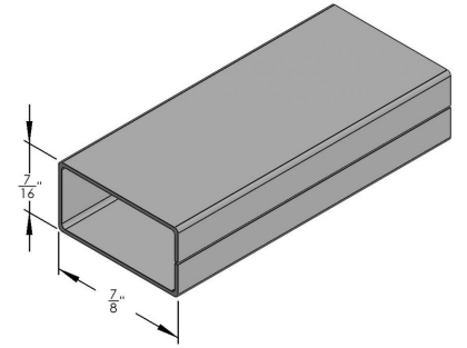
7/16 X 7/8 SDL GRILLE BAR - 152"
