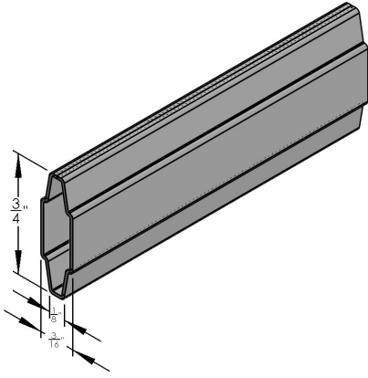
5.5MM X 18MM CONTOUR BAR - 12'8"
